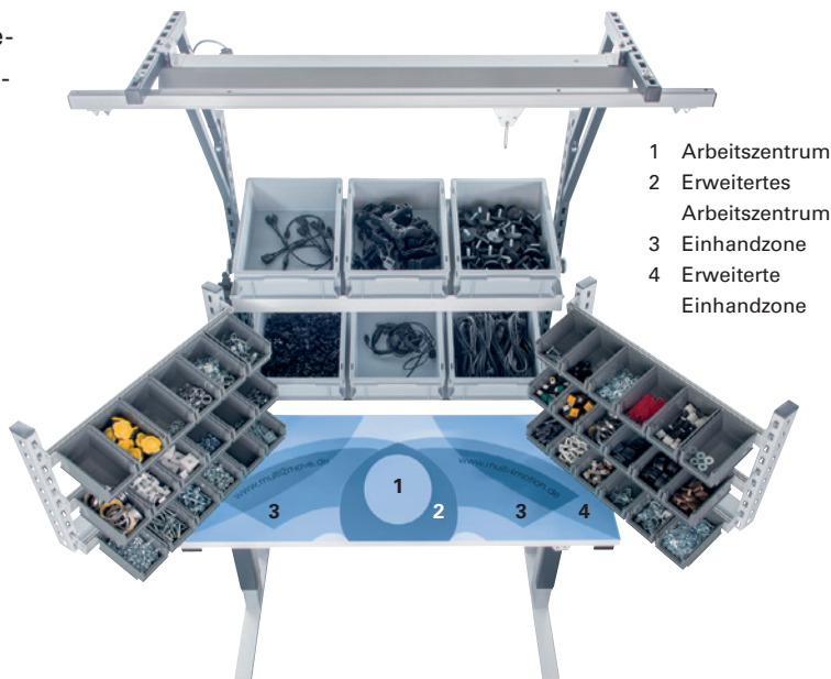
Ergonomischer Arbeitstisch mit Greifzonen-Übersicht
