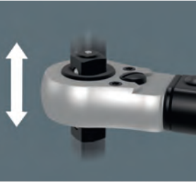
Durchsteckvierkant-Ausführung mit patentierter Nussverriegelung.
