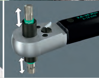
Beidseitige Bit-Aufnahme bei Rechts-/Linksanzug.
